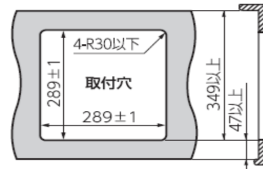
取付開口寸法
