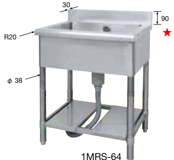
1槽丸脚前アール型シンク
