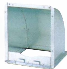
■ FFBDR-3HL-901 (W・BK) ※ ¥105,500 (900 × 605 × 600) ■ FFBDR-3HL-751 (W・BK) ¥79,600 (750 × 605 × 600) ■ FFBDR-3HL-601 (W・BK) ¥73,700 (600 × 605 × 600) 高さ700ミリも対応できます。 お問い合わせ下さい。
